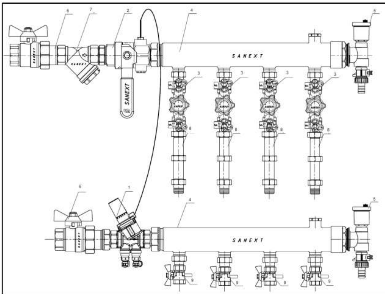
Рис. 2. Схема общая РКУ SANEXT Этажный
