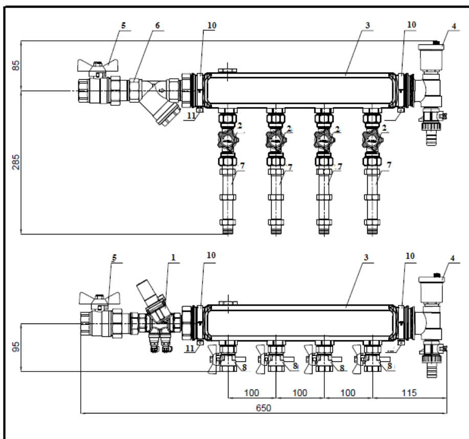
Рис. 3. Габаритные размеры PKV SANEXT Этажный на кронштейнах.
