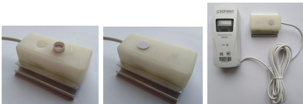
Рисунок 8 – Схема пломбировки распределителей тепла SANEXT-R-V
