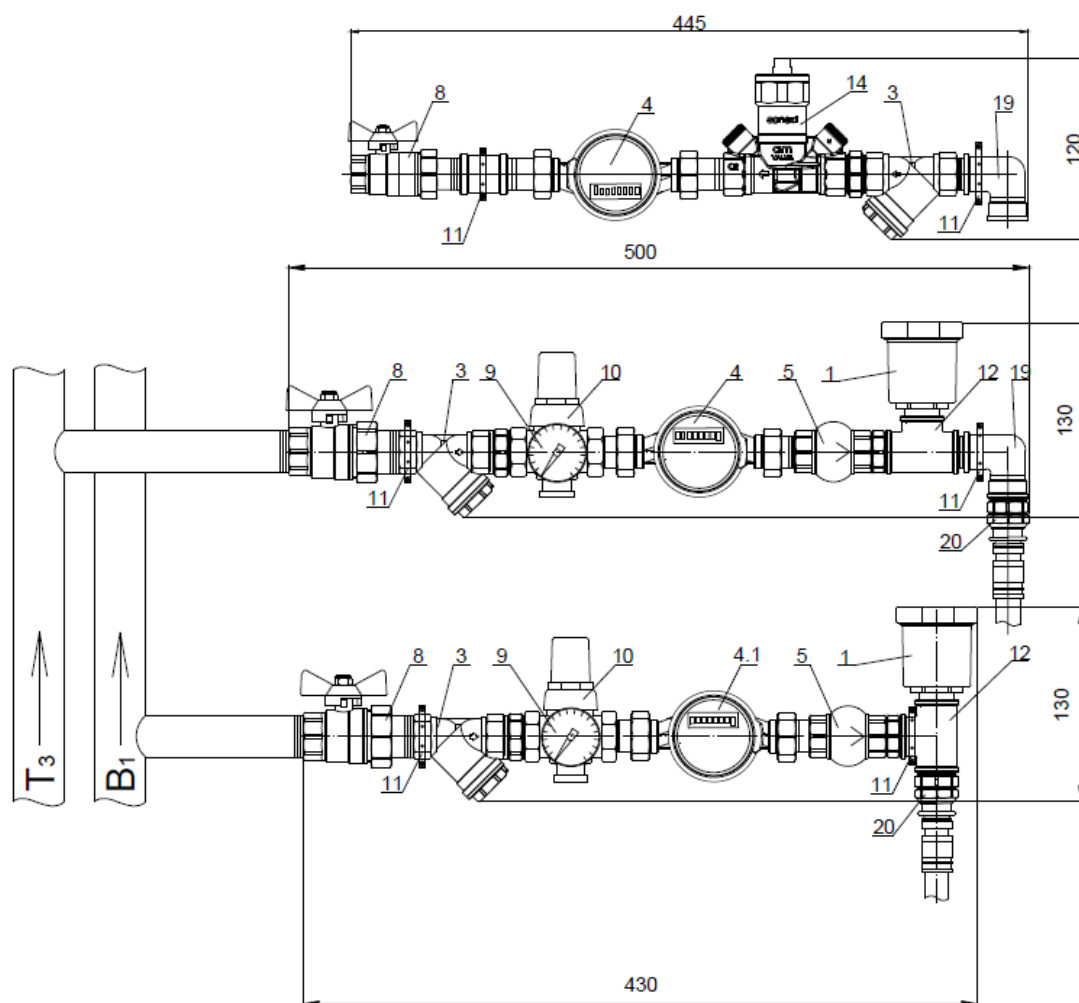
Рис. 3. Горизонтальное прямое исполнение (возможны отклонения размеров на 20-40 мм).
