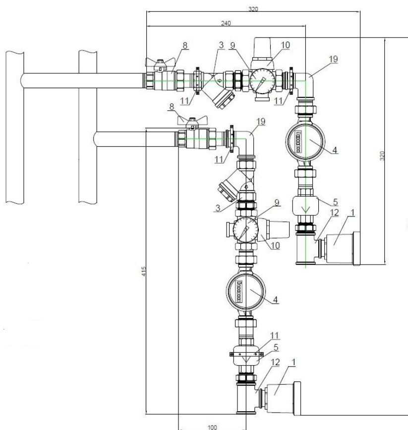
Рис. 4. Горизонтальное угловое исполнение.
