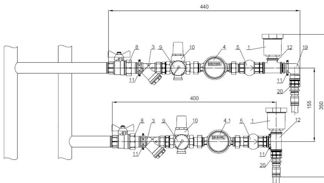
Рис. 3. Горизонтальное прямое исполнение.
