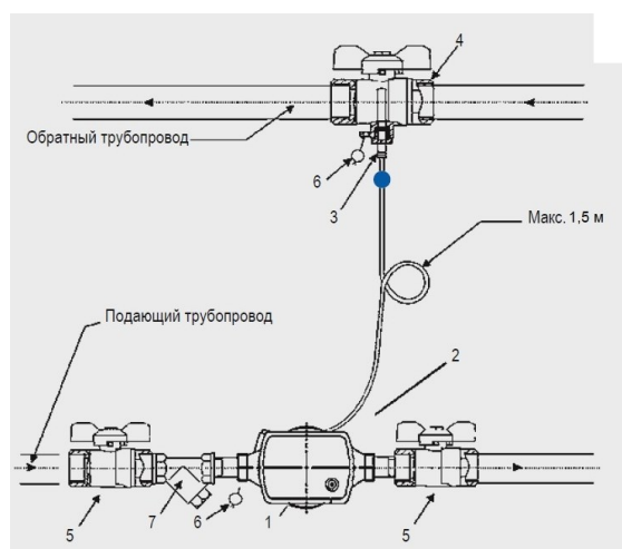
Рисунок 3 - Принципиальная схема общая подающий трубопровод
