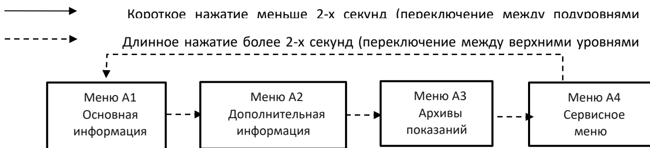
Рисунок 2– Схема меню верхнего уровня
