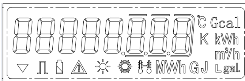
Рисунок 1 – Внешний вид дисплея теплосчетчика Sanext Mono CU
