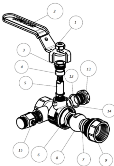
Рисунок 2. Шаровый кран ВВ для имп. трубки ДУ15-50 (арт 6301, 6302, 6303, 6304, 6305, 6306)
