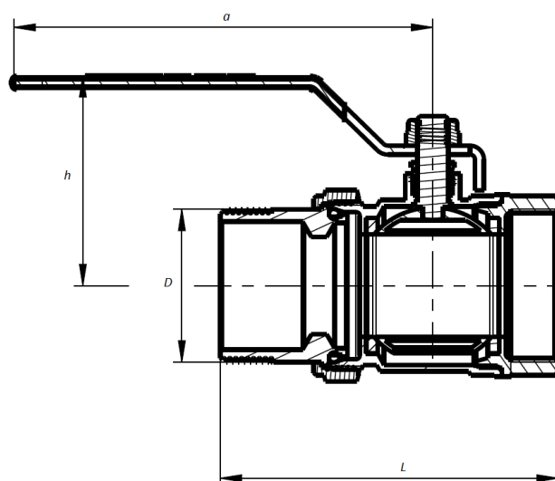
Рисунок 5 - Габаритные размеры арт. 8671, 8672, 8673, 8774, 8775, 8776
