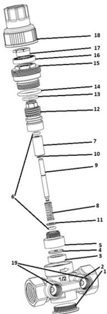
Рисунок 2- Комплектация ручного балансировочного клапана STP
