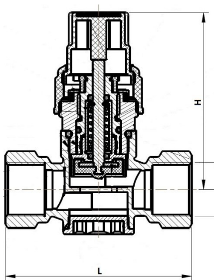
Рисунок 3 – Габаритные размеры клапана
