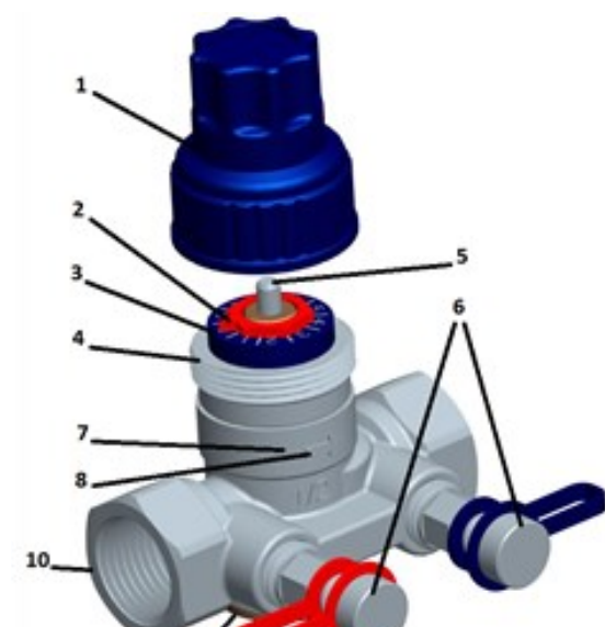
Рисунок 1 – Устройство ручного балансировочного клапана STP
