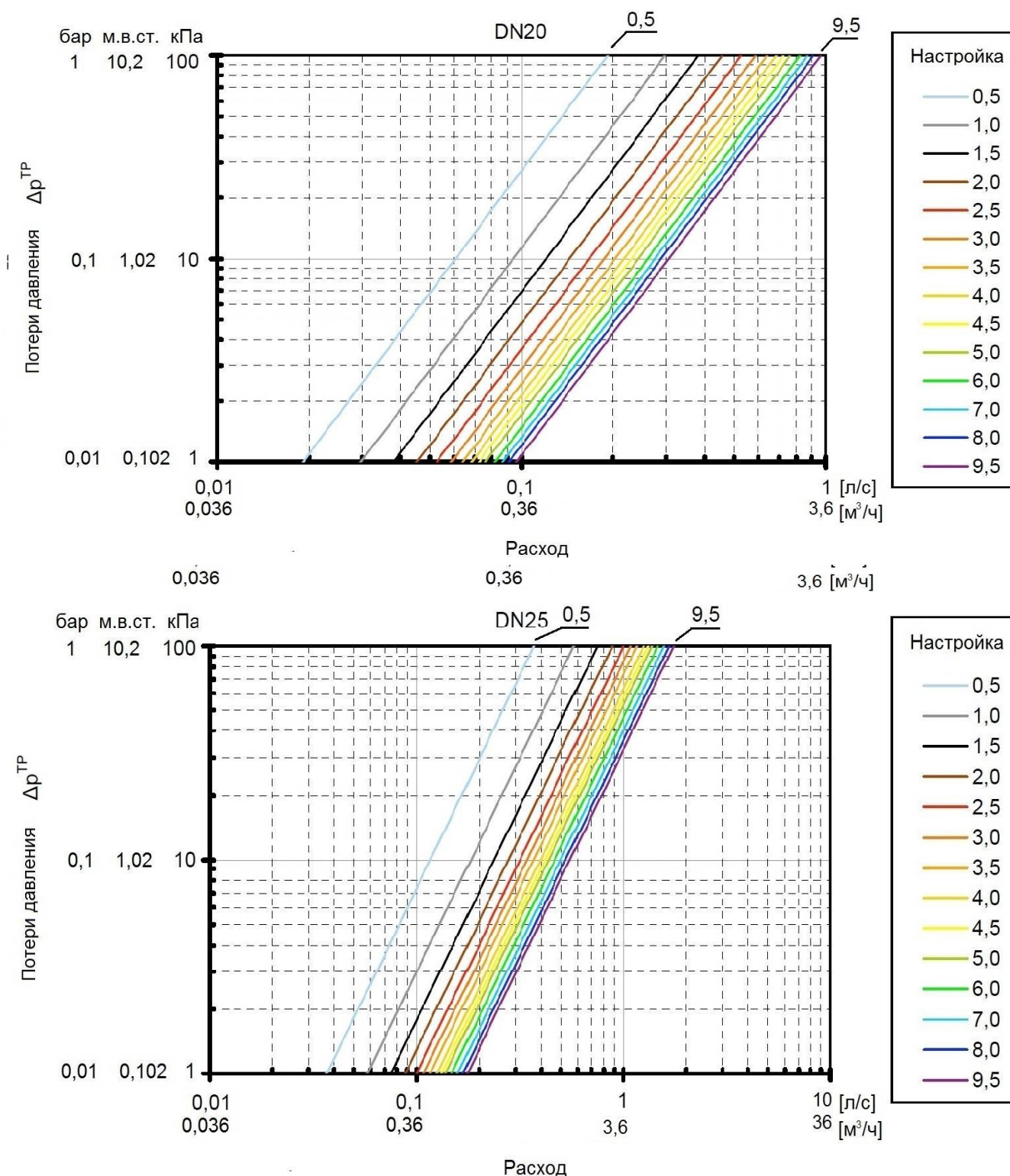
Рисунок 11 – График пропускной способности ручного балансировочного клапана STP
