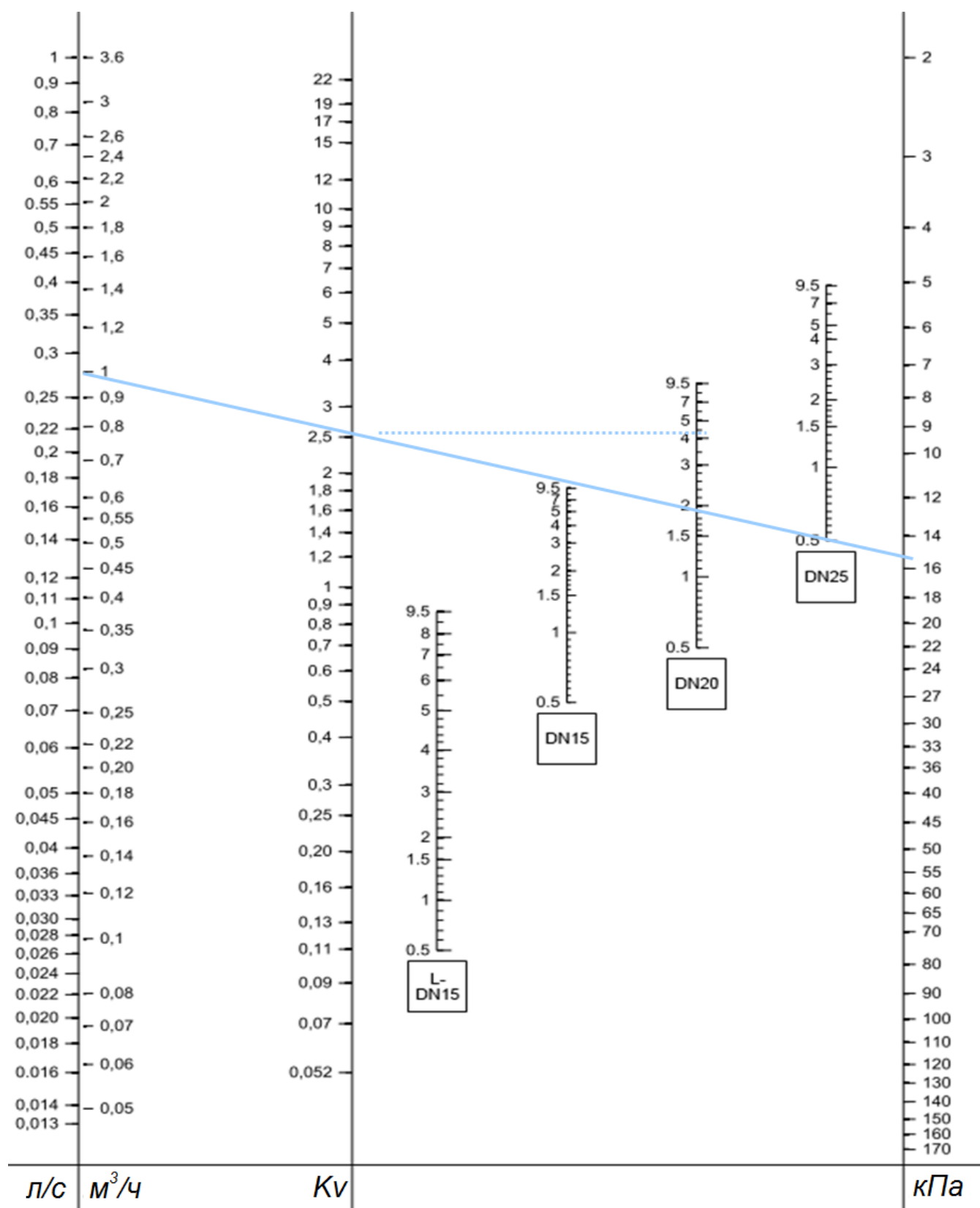
Рисунок 8 – Пример определения предварительной настройки клапана по диаграмме
