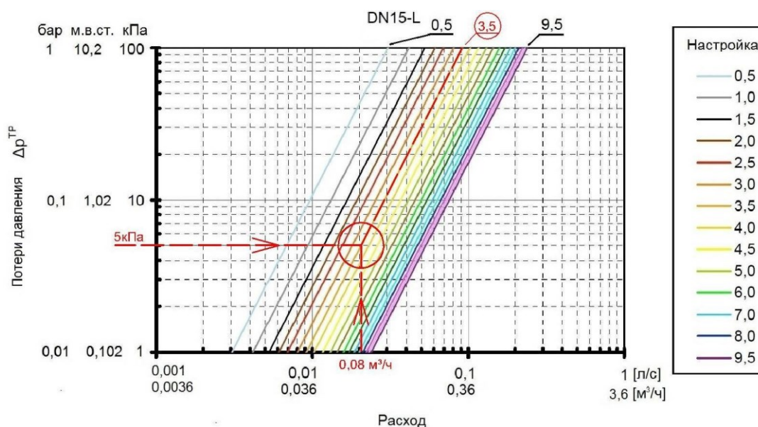
Рисунок 10 – Пример определения предварительной настройки клапана по графику
