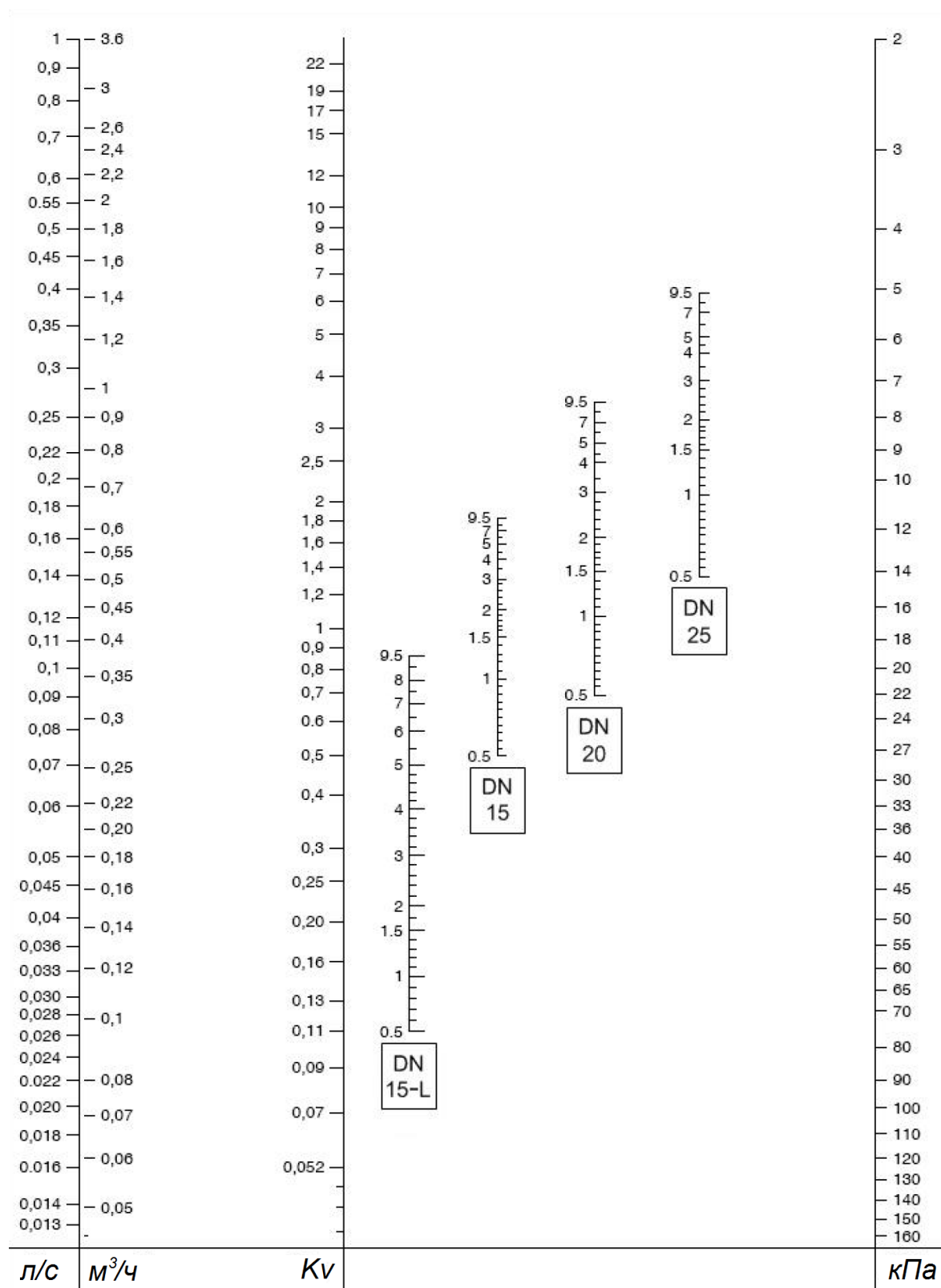
Рисунок 9 – Диаграмма значений предварительной настройки клапана
