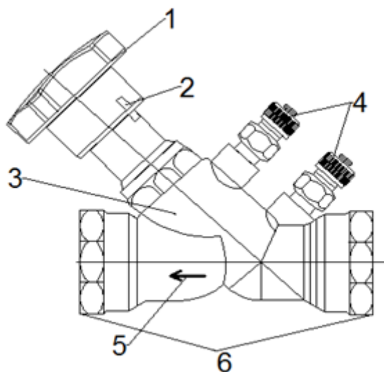
Рисунок 1 – Устройство ручного балансировочного клапана STP
