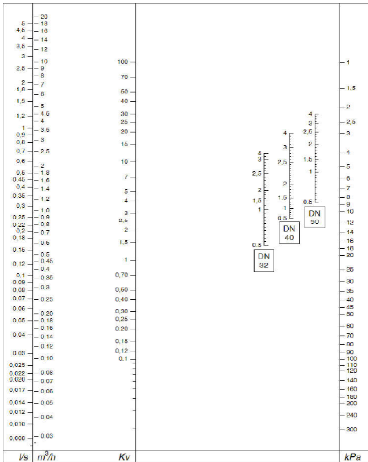
Рисунок 3 – Диаграмма настроек
