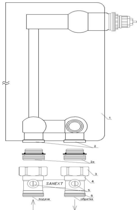
Рисунок 5- Схема подключения к радиатору с внутренней резьбой \frac{1}{2} " евроконус
