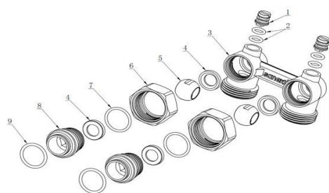
Рисунок 1 - Схема прямого узла нижнего подключения
