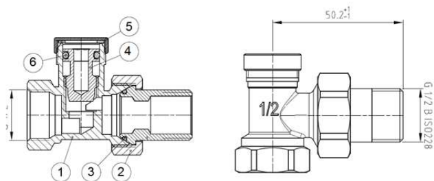
Рисунок 1 – Общая схема
