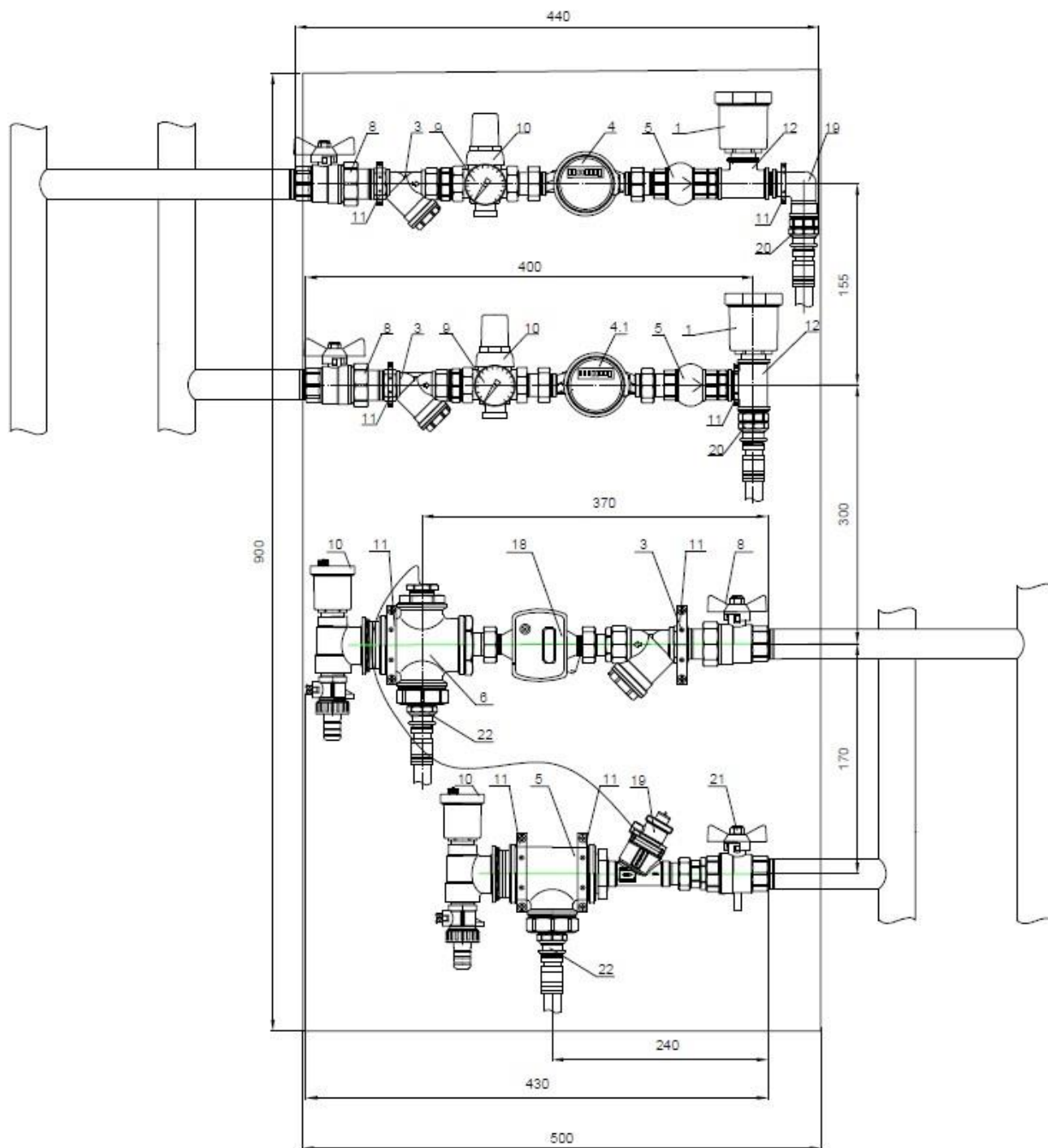
Рис. 3. Горизонтальное прямое исполнение.
