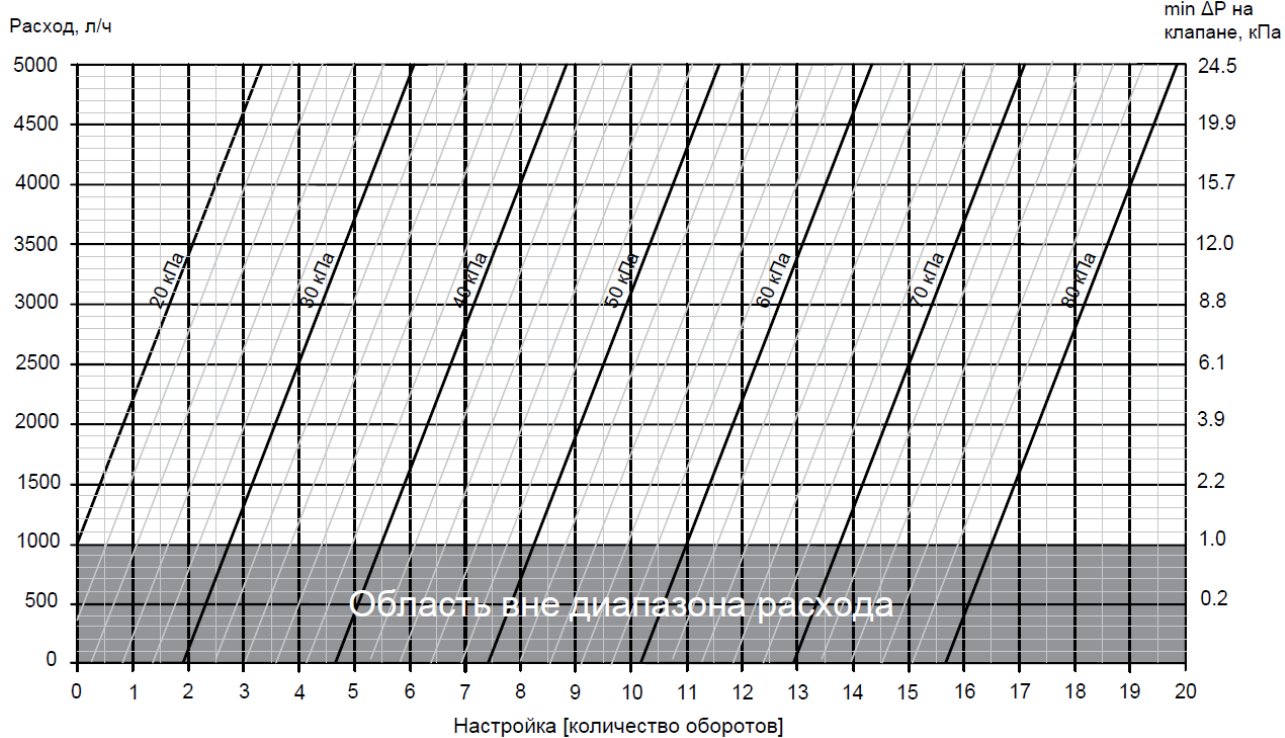
Рисунок 8. Автоматический балансировочный клапан SANEXT DPV DN 32.
