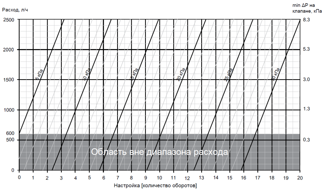
Рисунок 7. Автоматический балансировочный клапан SANEXT DPV DN 25.
