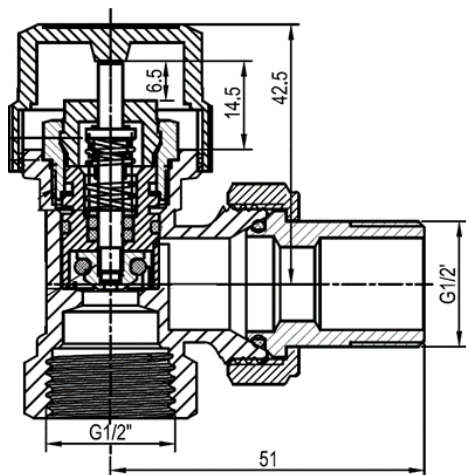
Рисунок 2 – Угловой клапан
