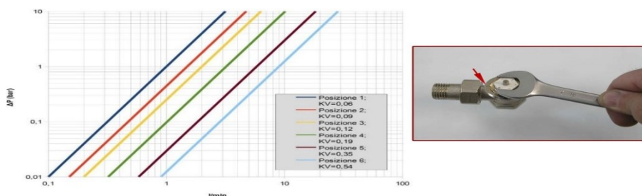
Рисунок 5 – Диаграмма настроечных значений
