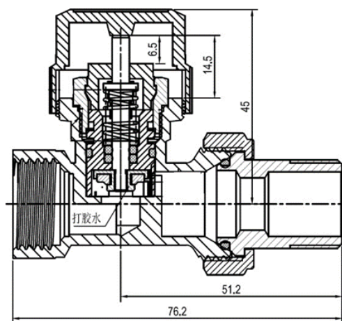
Рисунок 3 – Прямой клапан
