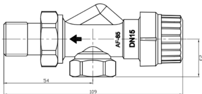
Рисунок 4 – Осевой клапан
