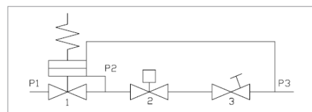
Рисунок 4 – Принцип действия клапана
