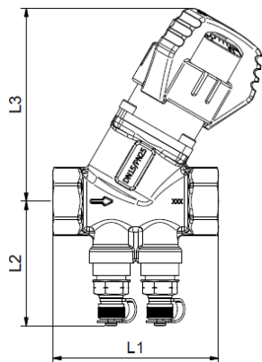
Рисунок 5 – Габаритные размеры
