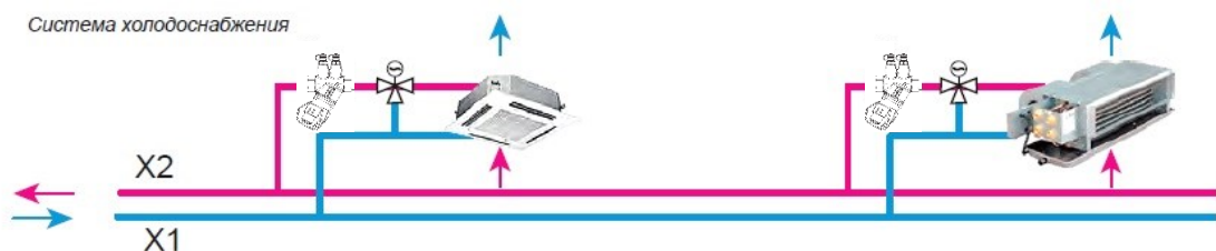
Рисунок 2 – Пример применения SANEXT FLV в обвязках фанкойлов, панелей лучистого обогрева или охлаждения и других вентиляционных установок в качестве автоматического балансирующего клапана – стабилизатора расхода.
