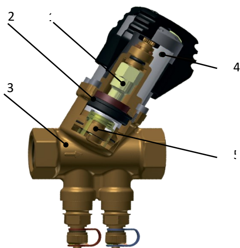
Рисунок 3 – Устройство клапана
