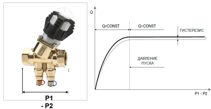
Рисунок 6 – График перепада давления
