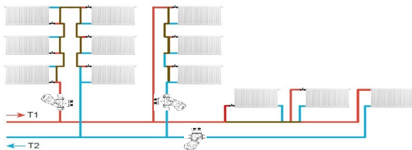
Рисунок 1 - Пример применения SANEXT FLV на стояках однотрубной системы отопления
