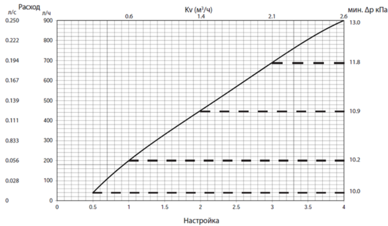
Рисунок 7 – График пускового значения перепада давления от выставленной преднастройки FLV DN 15
