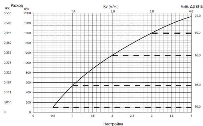
Рисунок 8 – График пускового значения перепада давления от выставленной преднастройки FLV DN20
