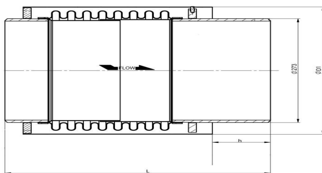
Рисунок 2 – Габаритные размеры сильфонных компенсаторов ДУ 65-250 мм
