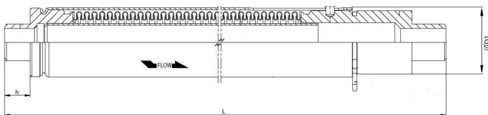
Рисунок 1 – Габаритные размеры сильфонных компенсаторов Ду 15-50 мм
