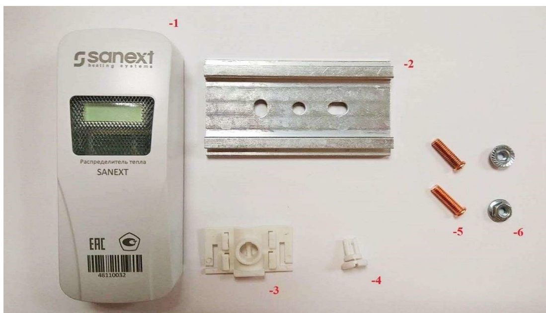
Рисунок 5 – Комплектация распределителя тепла SANEXT и монтажного комплекта для крепления на панельные радиаторы Порядок действия:
