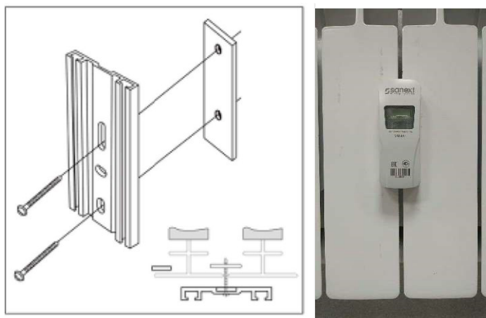
Рисунок 4 – Установка на секционный радиатор
