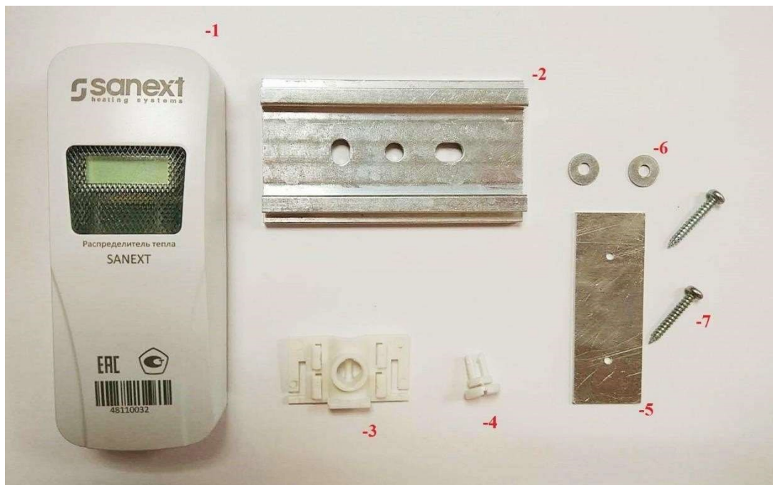
Рисунок 3 – Комплектация распределителя тепла SANEXT и монтажного комплекта для крепления на биметаллические или алюминиевые секционные радиаторы
