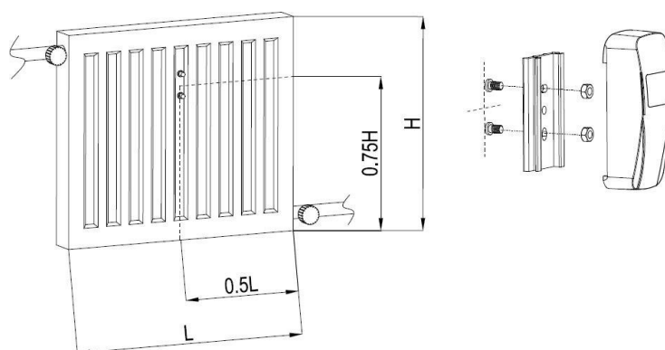
Рисунок 6 – Установка на панельный радиатор
