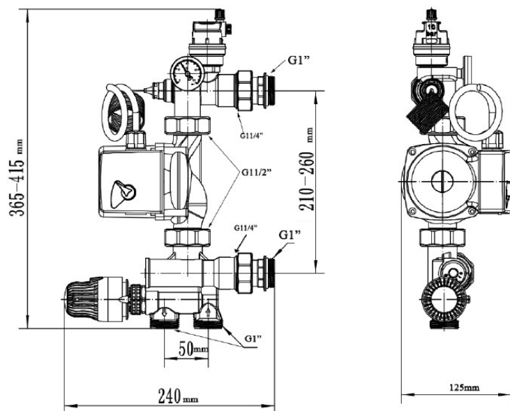
Рисунок 1 – Габаритные размеры 5
