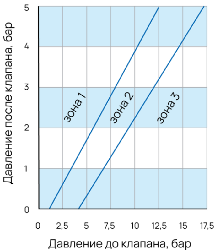
Рисунок 3 – График кавитации
