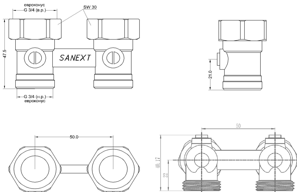
Рис. 1. Схема общая 2 .
