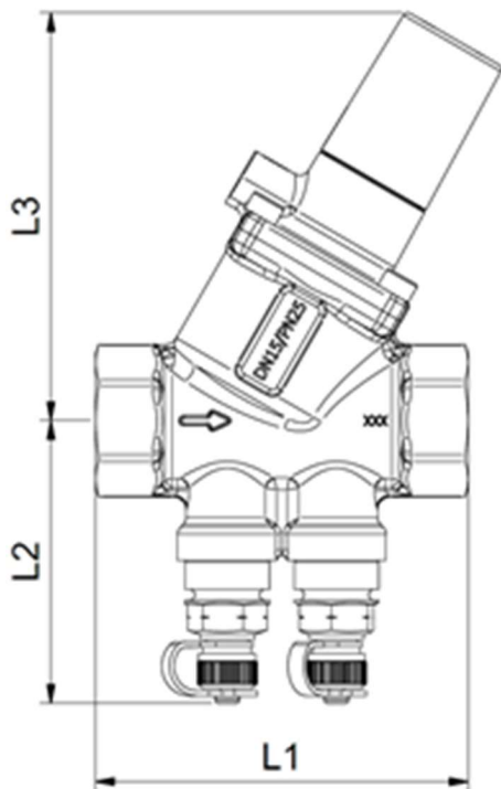
Рисунок 2. Габаритные размеры DPV
