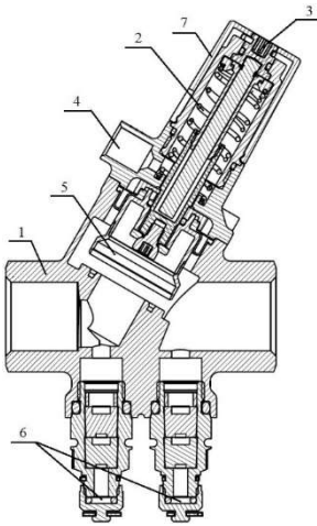
Рисунок 1. Устройство клапана DPV.
