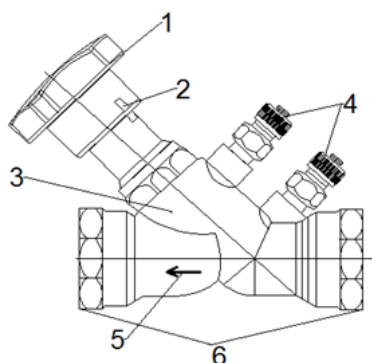
Рисунок 1 – Устройство ручного балансировочного клапана STP
