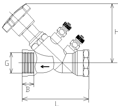
Риснок 2 – Габаритные размеры
