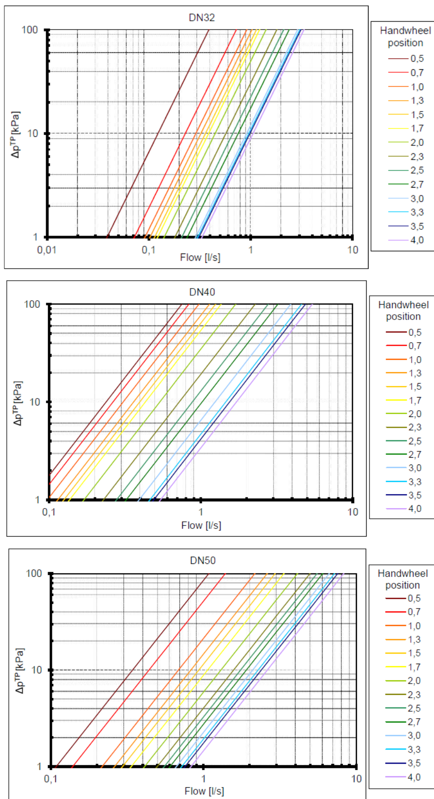
Рисунок 7 — Графики пропускной способности
