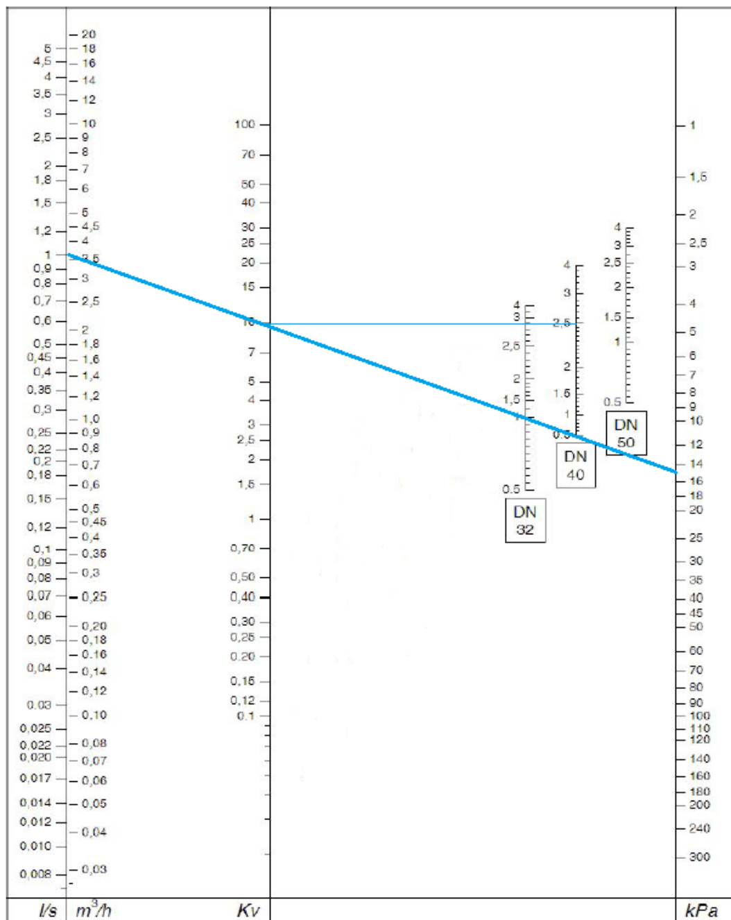
Рисунок 5 – Диаграмма значений предварительной настройки клапана
