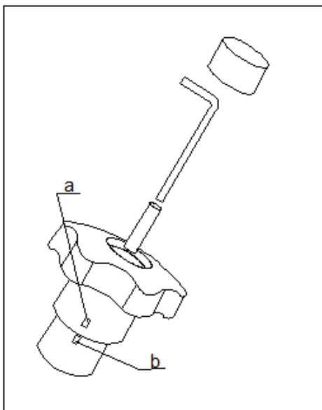
Рисунок 4 – Пример гидравлической настройки
