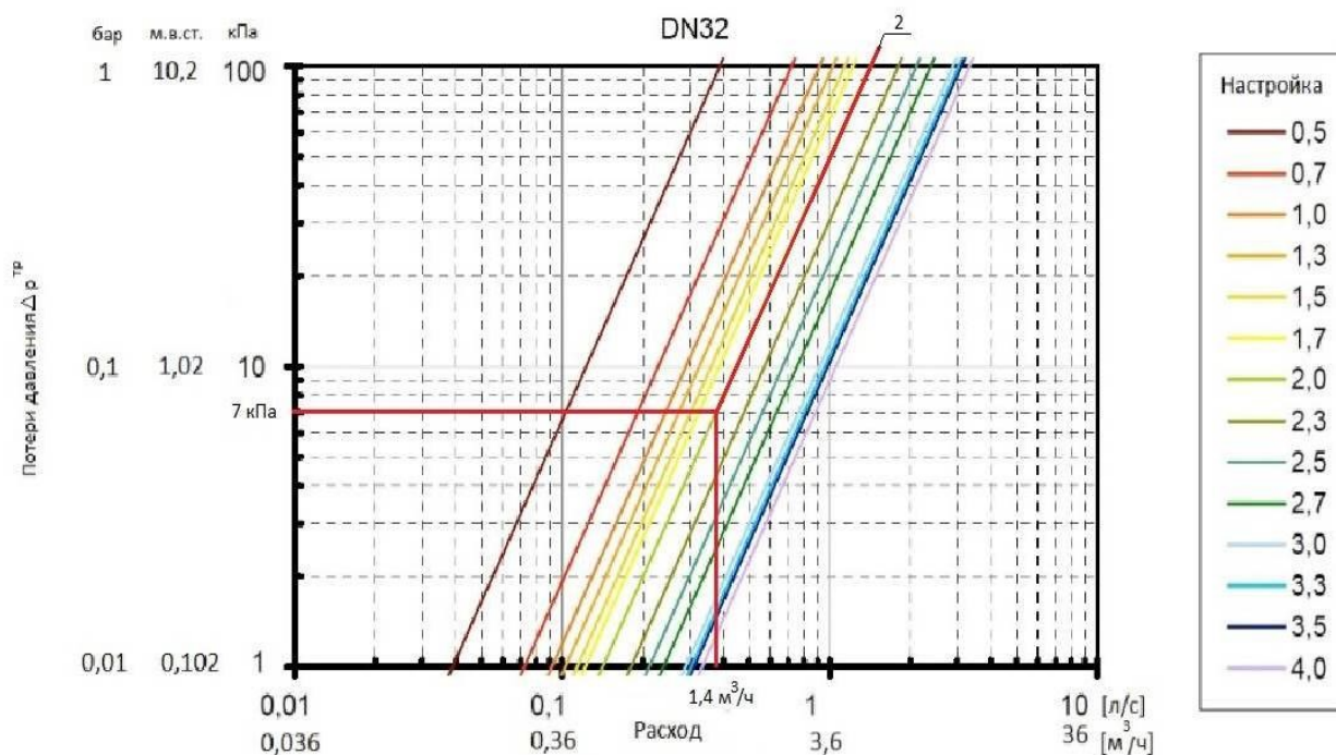
Рисунок 6 – Пример определения предварительной настройки клапана по графику
