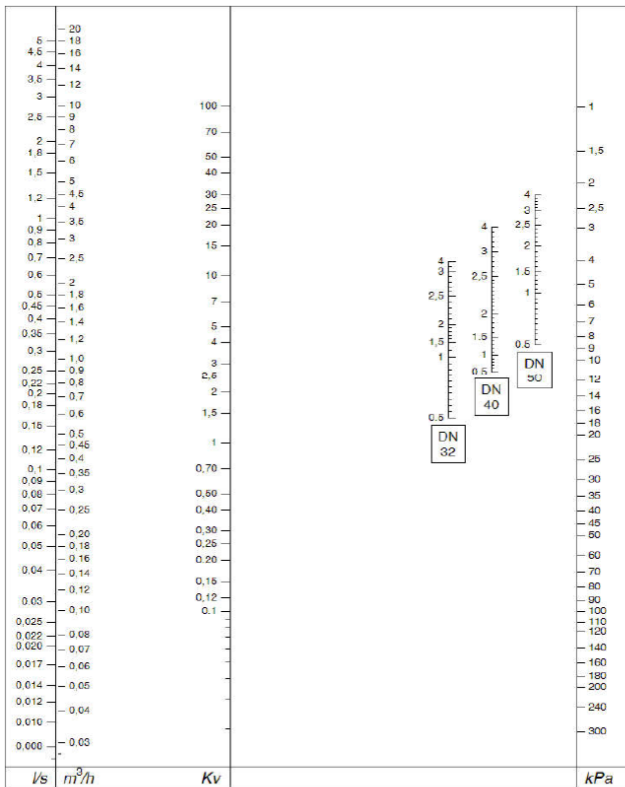
Рисунок 3 – Диаграмма настроек
