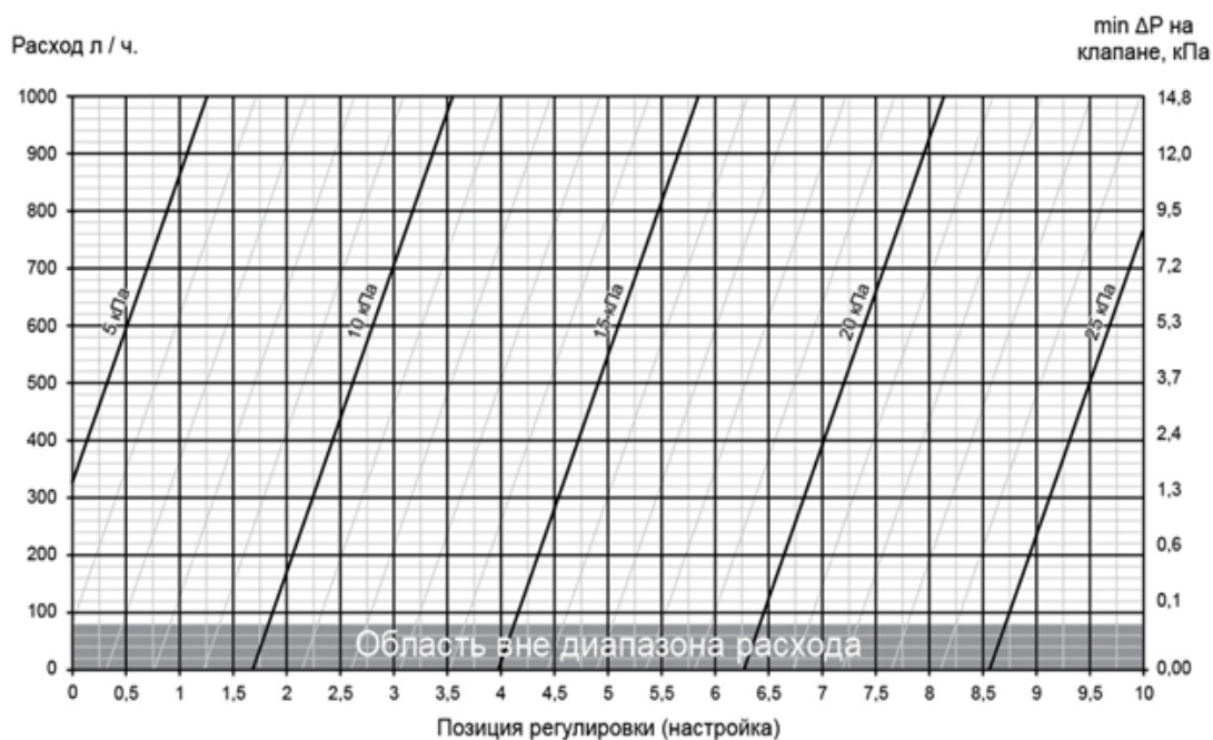
Рисунок 4 – График расхода
