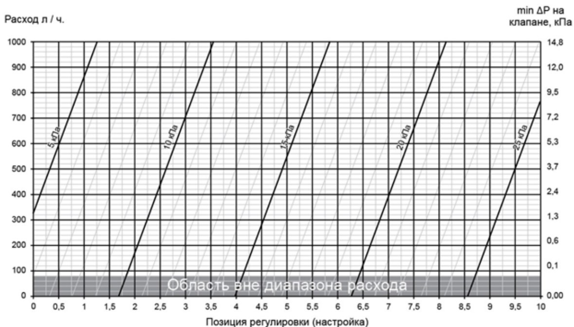
Рисунок 3 – График предварительной настройки клапана
