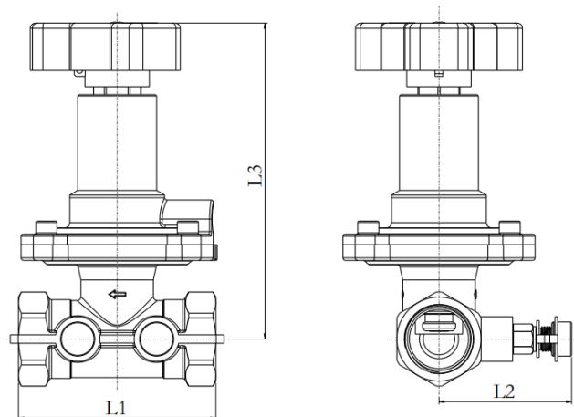
Рисунок 2 – Габаритные размеры
