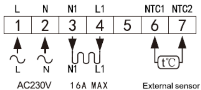
Рисунок – 3. Схема подключения
