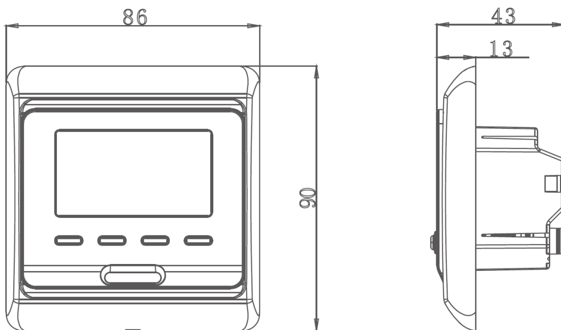
Рисунок – 2. Габариты
