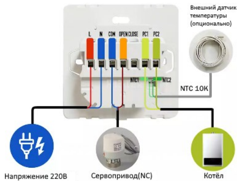
Рисунок 3 – Пример подключения №1
