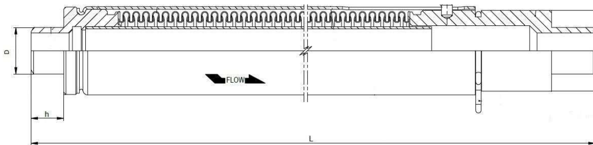
Рисунок 2 – Осевой сифонный компенсатор Ду 15-50 мм
