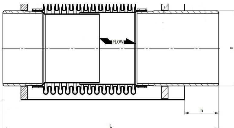
Рисунок 3 – Осевой сифонный компенсатор Ду 65-150 мм
