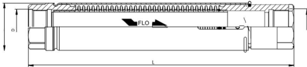
Рисунок 1 – Габаритные размеры сильфонного компенсатора
