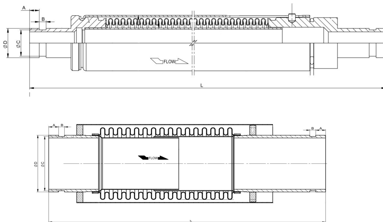
Рисунок 4 - Габаритные размеры сиффонных компенсаторов Ду 15-50 мм и Ду65 -200 мм
