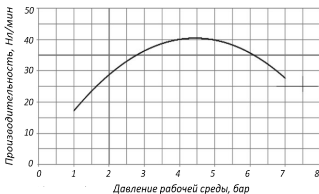
Рисунок 2 – График производительности
