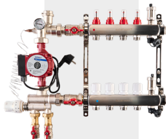
ПКУ SANEXT «Тёплый пол» с насосно-смесительным узлом MU-S
