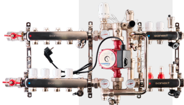
ПКУ SANEXT «Тёплый пол» с насосно-смесительным узлом MU-C
