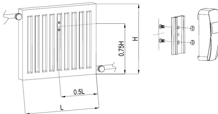
Рис. 6 Установка на панельный радиатор
